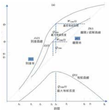
▲圖2 道路車輛累積到達與離開／紓解曲線圖
